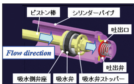
図4 ユニフロー式ポンプの構造
