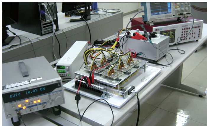
写真3 熱電素子によって作られた数十ボルトの直流電圧を家庭用の交流100ボルトに昇圧するための実験。変換に伴う損失を電力アナライザーで測定し、損失を低減する回路を研究している
