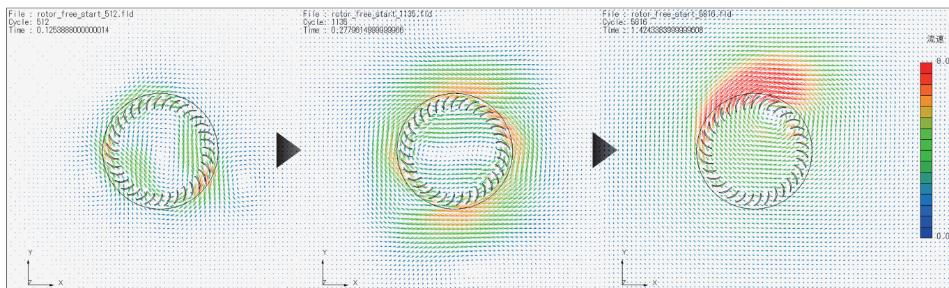
図3 クロスフローファンを単独で回した場合の流れ場の変化 はじめに円筒外に出ていく複数の流れが起こるが、やがてそれらは合体して1つになり、周囲をファンの回転速度より遅い速度で回る
